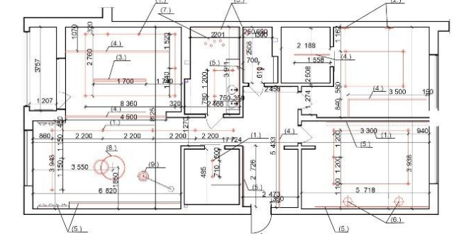
ПЛАН ПОТОЛКОВ СО СВЕТИЛЬНИКАМИ
