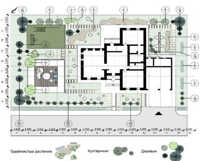
ДЕНДРОПЛАН М 1:200
