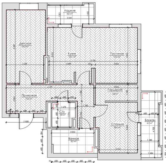
План раскладки напольных покрытий
