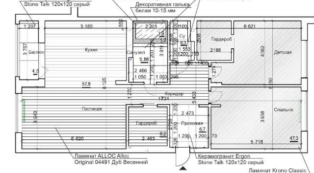
ПЛАН ПОЛОВ
