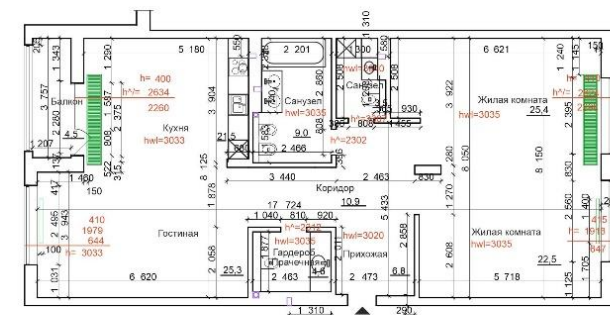
ПЛАН ДО ПЕРЕПЛАНИРОВКИ
