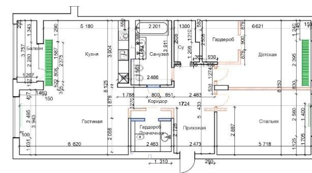
ПЛАН ПЕРЕПЛАНИРОВКИ
