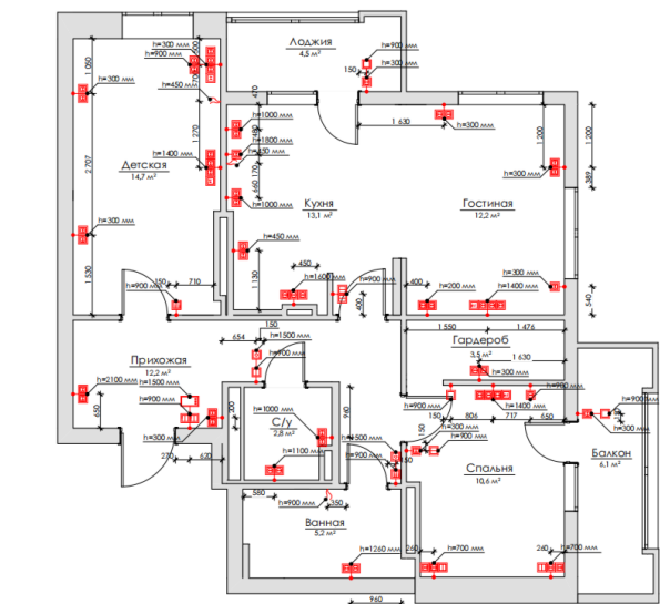
План электрики (розетки и выключатели)
