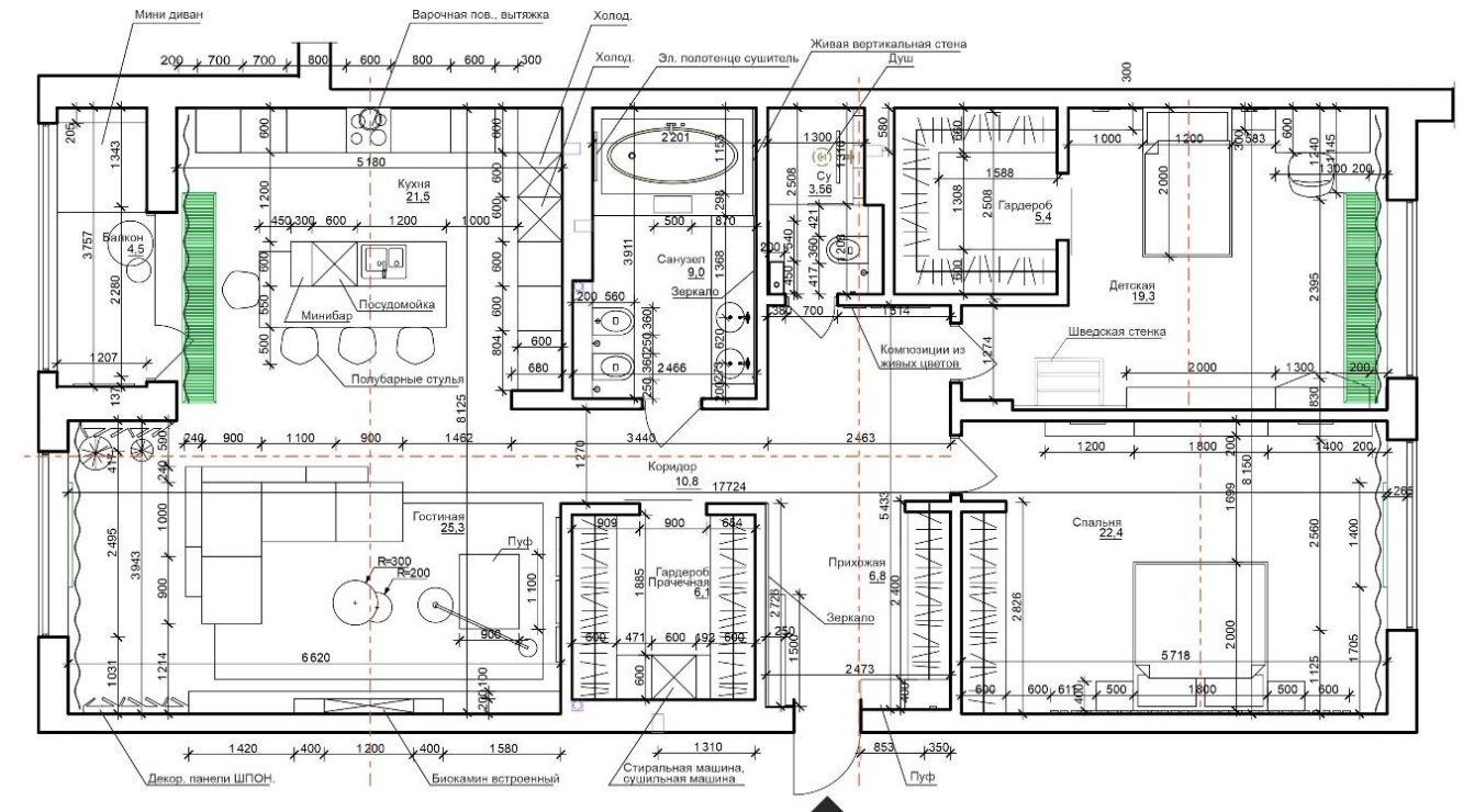
ПЛАН ДО ПЕРЕПЛАНИРОВКИ
