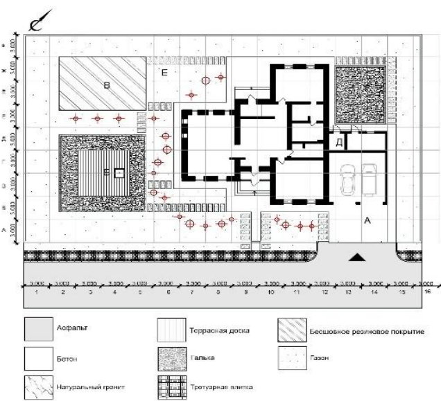
ПЛАН ПОКРЫТИЙ М 1:200
