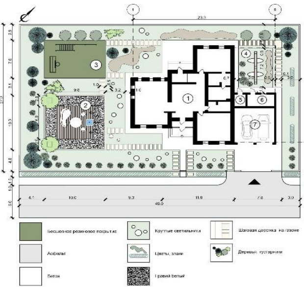
СХЕМА ГЕНПЛАН М 1:200
